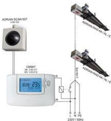
Prípojenie plynových infražiaríčov k týždennému programovateľnému termostatu CM907
