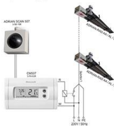
Prípojenie plynových infražiaríčov k týždennému programovateľnému termostatu CM507
